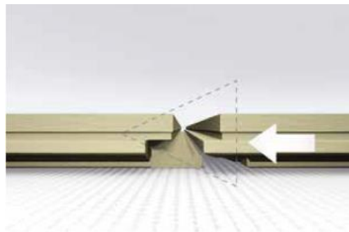
Горизонтальное соединение
